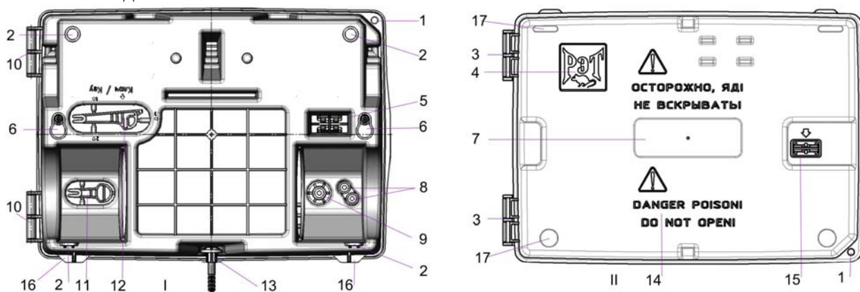
Корпус - вид снизу (I), крышка - вид сверху (II)
